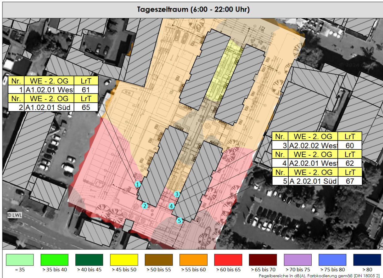
Abbildung 9: Rasterlärkarte für die Außenwohnbereiche, Immissionshöhe 2. OG, Straßenverkehr
