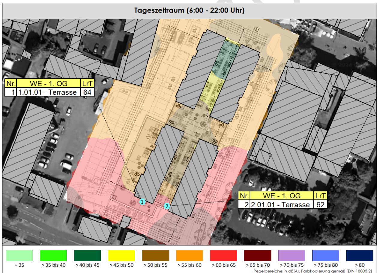
Abbildung 8: Rasterlärmkarte für die Außenwohnbereiche, Immissionshöhe 1. OG, Straßenverkehr
